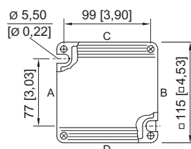
8118/1.2. Enclosure SZ 2
