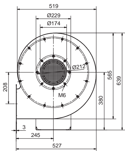
Ansicht A View A
